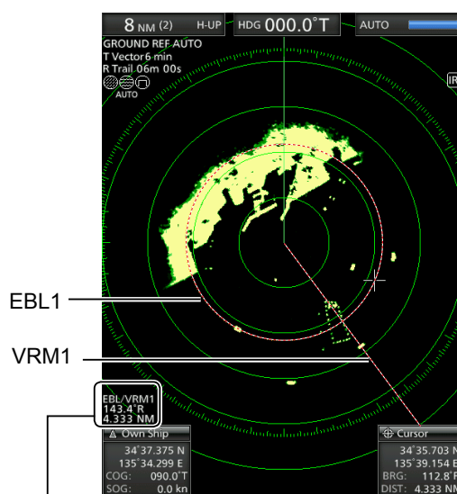
EBL/VRM1 readout
