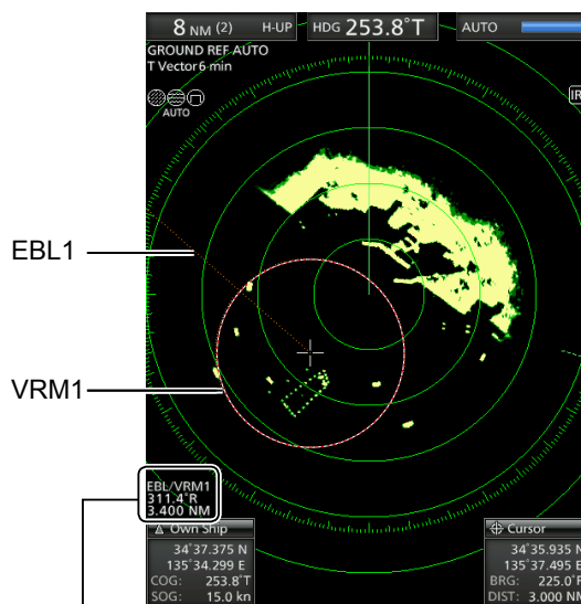
EBL/VRM1 readout
